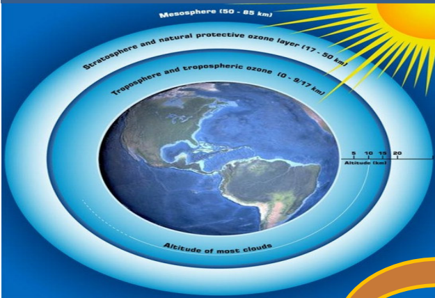
CAMADA DE OZÔNIO (O 3 )
